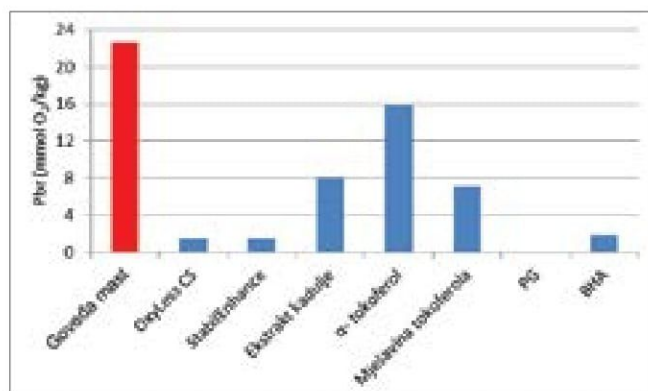
Grafikon 2. Utjecaj antioksidanasa na oksidacijsku stabilnost govedjeg loja nakon 120 sati testa održivosti Graph 2 Influence of antioxidants on the oxidative stability of beef tallow after 120 hours of sustainability test.
